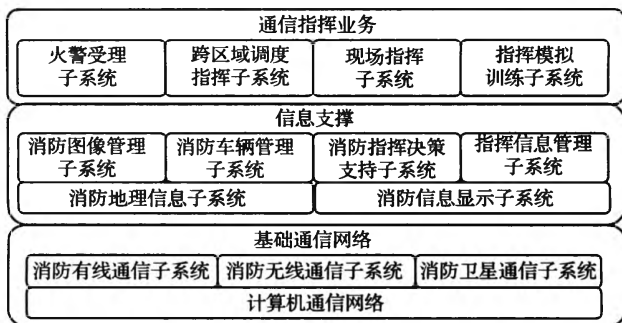
图 3.0.2 消防通信指挥系统的技术构成
